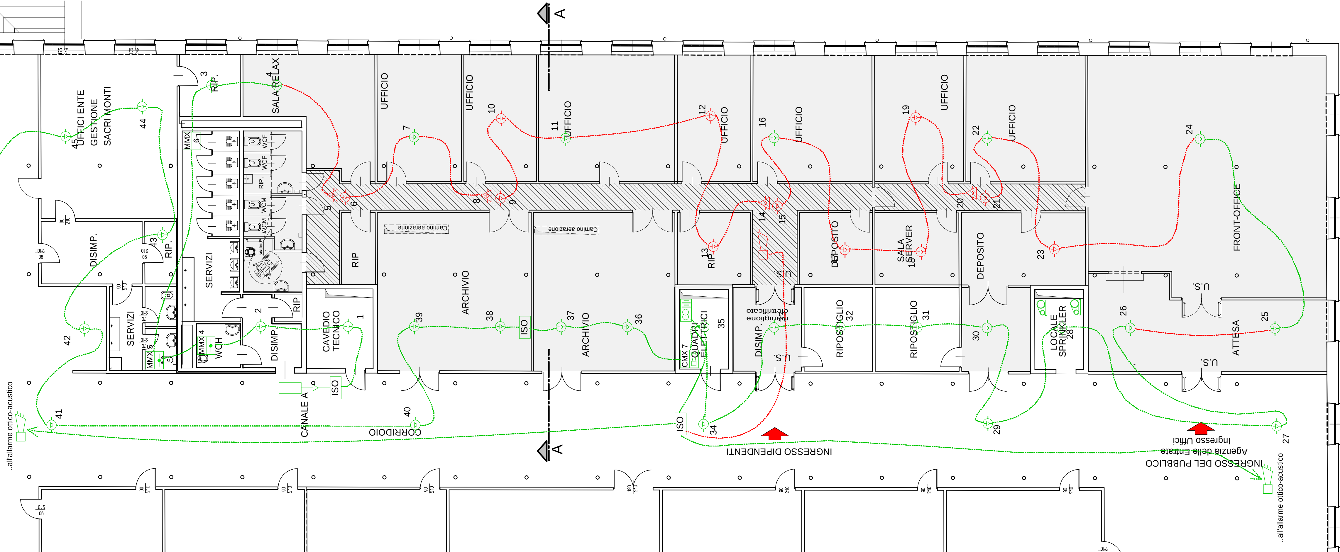
IMPIANTO RIVELAZIONE INCENDI A SOFFITTO PROGETTO - Scala 1.100
